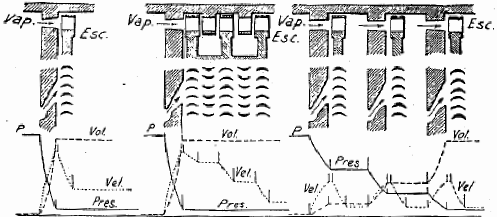
Turbina de acción Curtis Etapas de Velocidad
